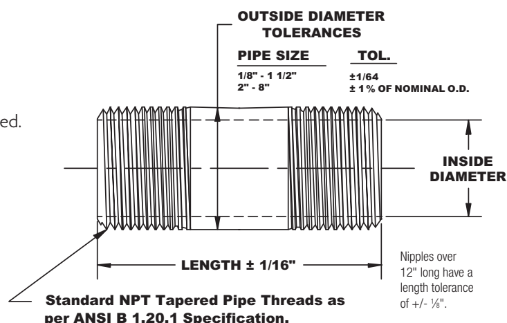
FIG. 335: Extra Heavy Galv. Sch. 80
